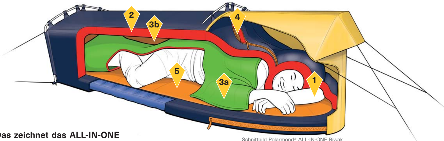
Schnittbild Polarmond® ALL-IN-ONE Biwak
